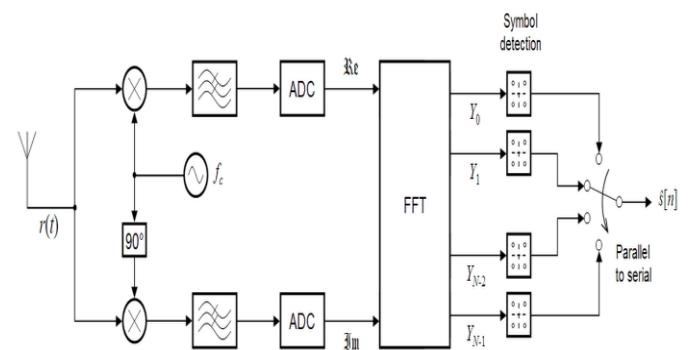
Fig: 4 RECIVER
